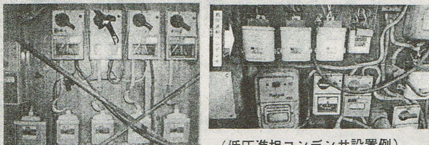
(低圧進相コンデンサ設置例)
